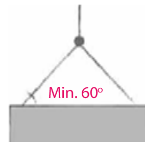
Figur 8: vinkel på løftekæder
