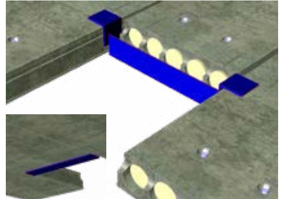
Figur 4: Standard udvekslingsbjælke (UVB)
